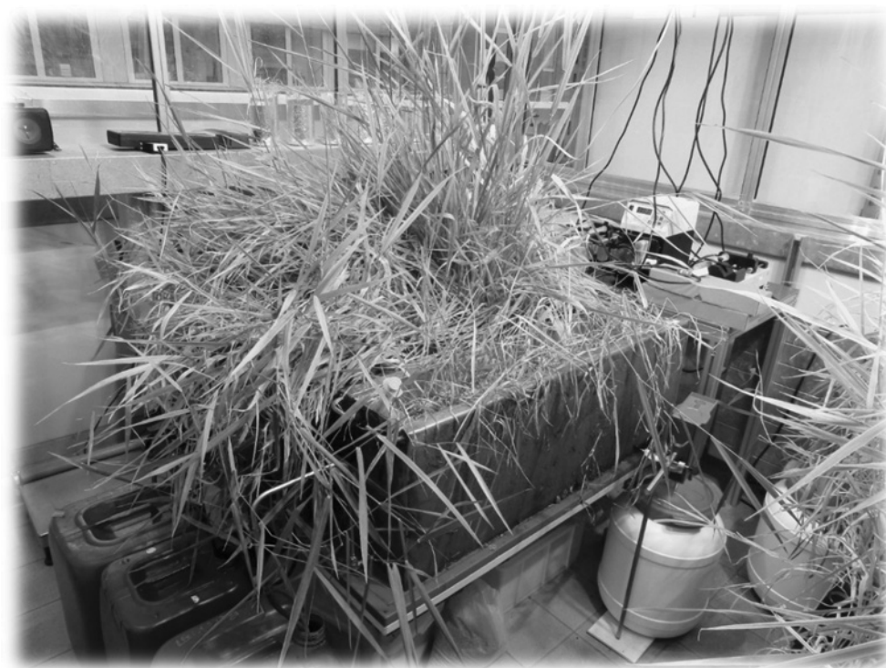
Рис. 3. Экспериментальная установка
